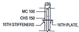
DETAIL-B
